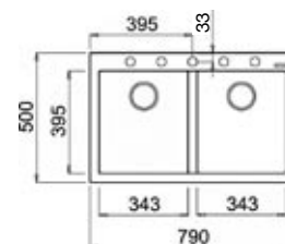
QUADRA 350 cm. 79x50 (2 v. prof. 21) (foro incasso 77x48)
