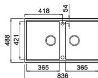
BEST 450 cm. 83,6x48,8 (2 v. prof. 20) Sottotop (foro incasso sottotop 79,5x44,8)
